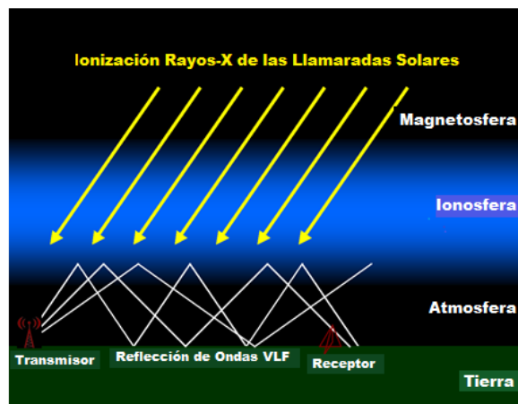
La ionosfera de la Tierra y el suelo forman una "guía de ondas" a través de la cual las señales de radio VLF se propagan o "rebotan" en torno a la Tierra. Imagen cortesía de Morris Cohen, Universidad de Stanford
