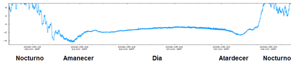
Ejemplo de gráfica de datos SID
