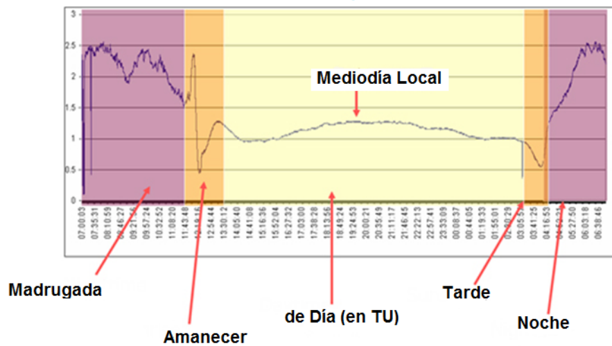
Muestra de datos SID diaria (colores añadidos)
