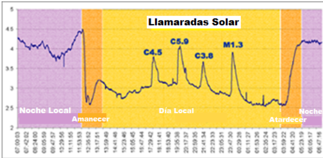
Gráfica de datos de SID (se añaden colores y etiquetas para mayor claridad)
